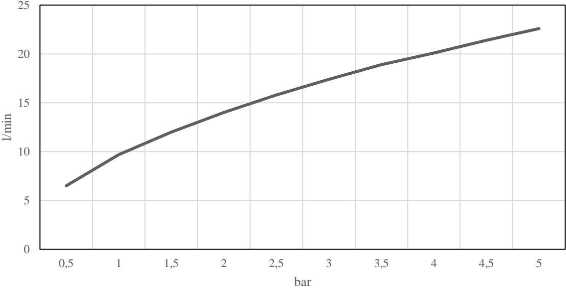
QS3300 flow rate(l/min)
